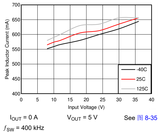
图 6-6. I_{PEAK-MIN}
