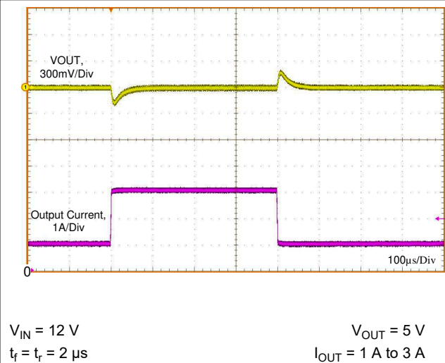
图 9-24. Load Transient
