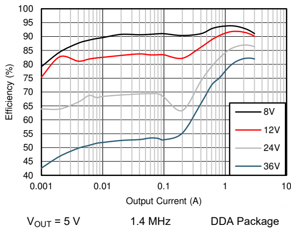
图 9-9. Efficiency
