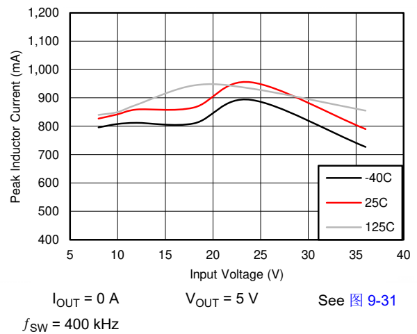
图 7-6. I_{PEAK-MIN}
