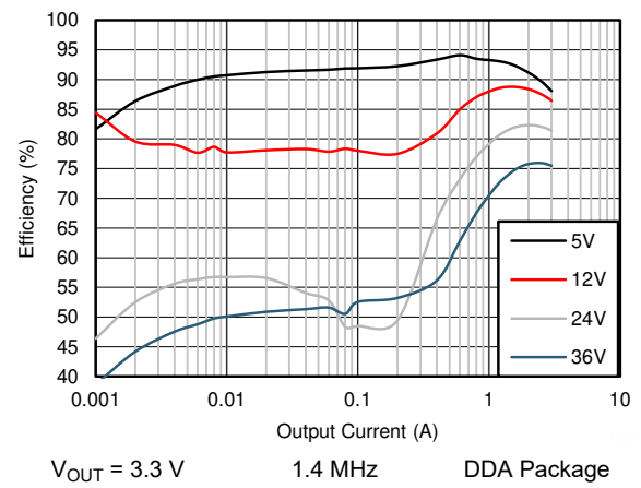
图 9-10. Efficiency
