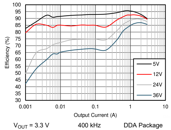
图 9-8. Efficiency
