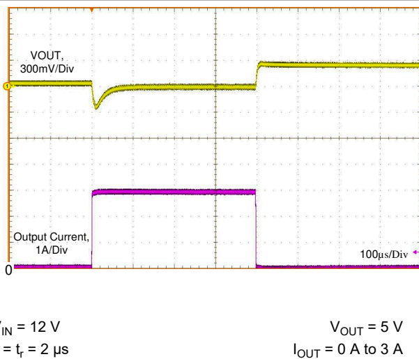
图 9-23. Load Transient
