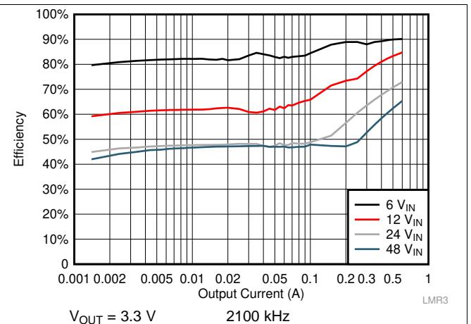
图 44. Efficiency
