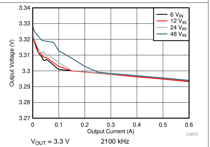
图 46. Load Regulation
