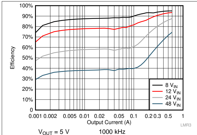
图 21. Efficiency
