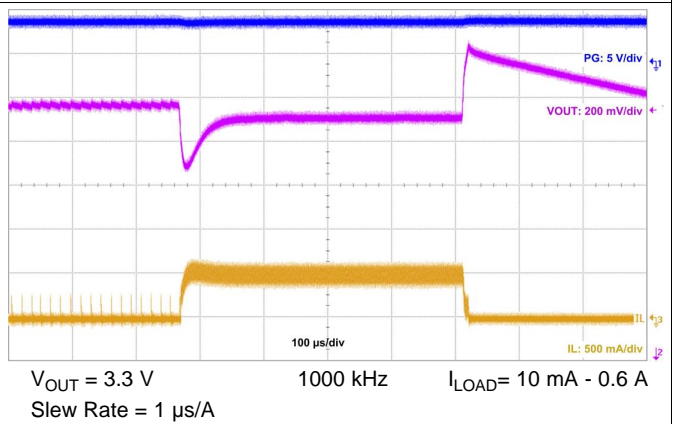
图 32. Load Transient
