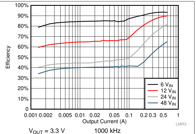
图 22. Efficiency
