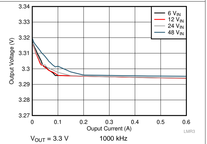
图 24. Load Regulation
