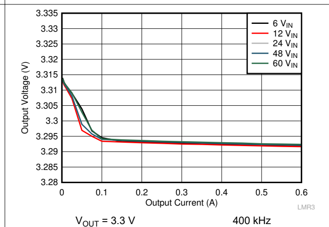
图 9-8. Load Regulation
