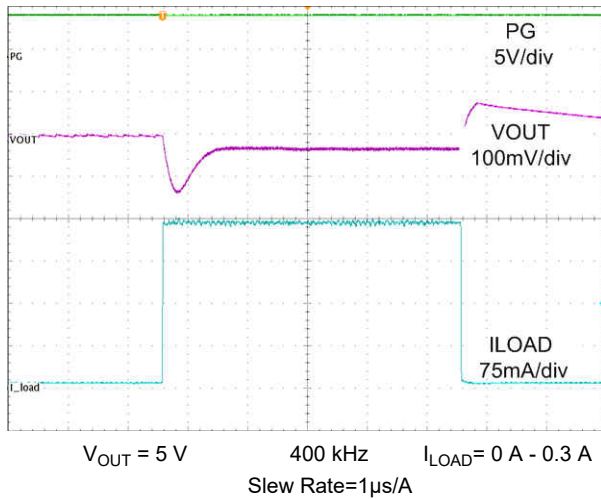
图 9-15. Load Transient
