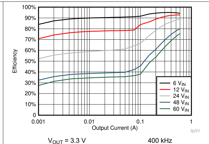
图 9-6. Efficiency
