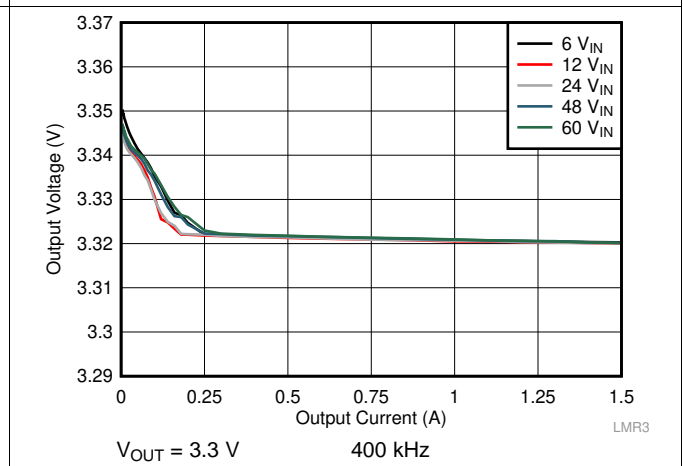
图 25. Load Regulation
