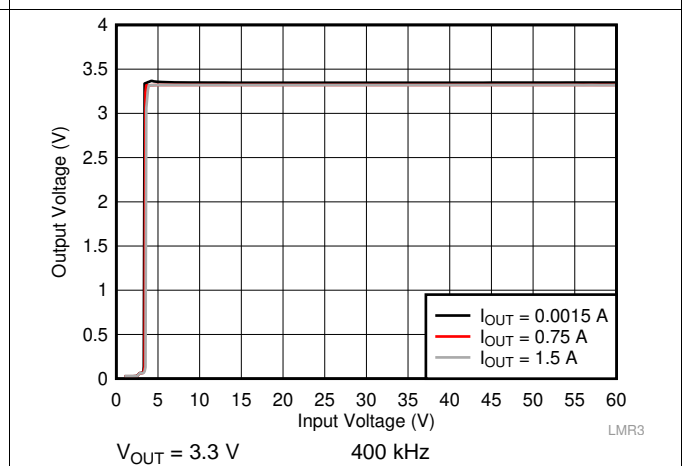
图 27. Line Regulation
