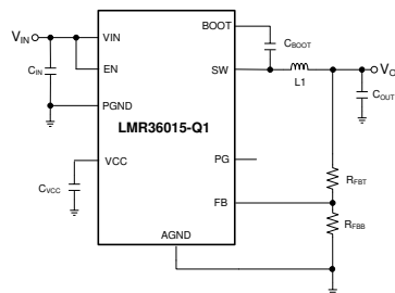
简化原理图
