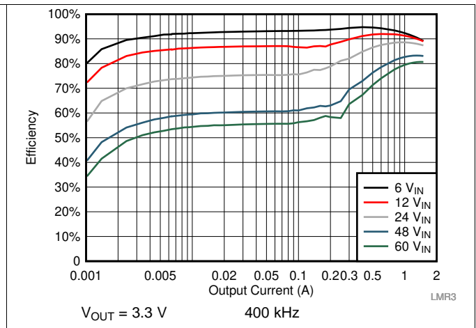
图 23. Efficiency
