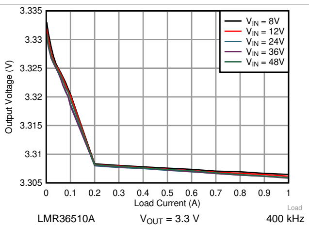
图 17. Load Regulation
