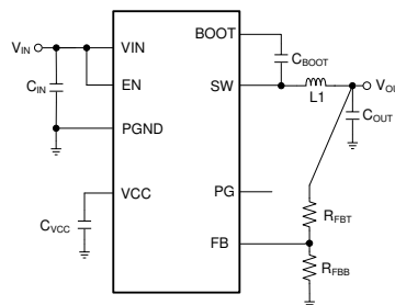
简化原理图
