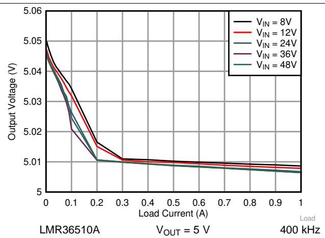
图 19. Load Regulation
