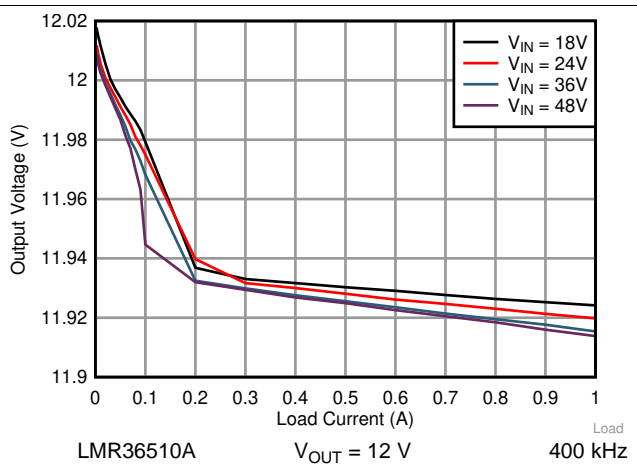
图 21. Load Regulation
