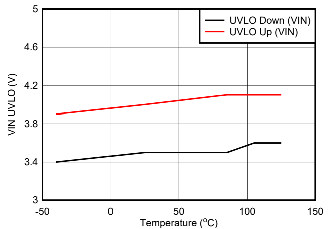
图 7-6. V_{IN} UVLO vs Temperature
