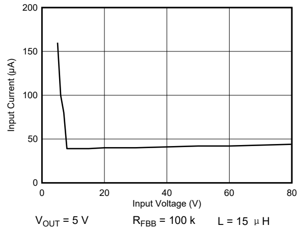
图 7-2. No Load Input Current vs Input Voltage
