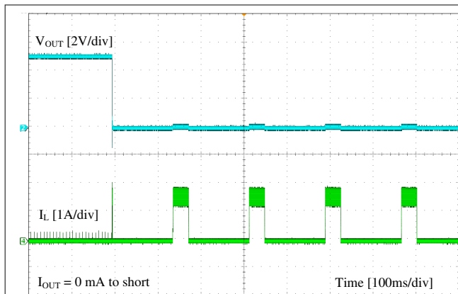
图 9-9. Short Protection
