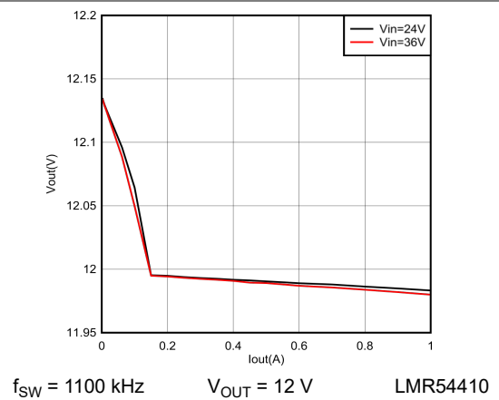
图 7-8. 12-V Load Regulation
