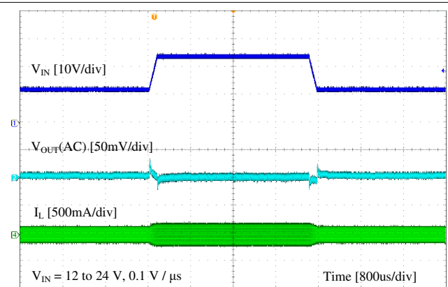
图 9-8. Line Transient
