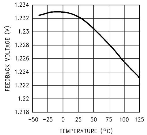
反馈电压与温度的关系曲线
