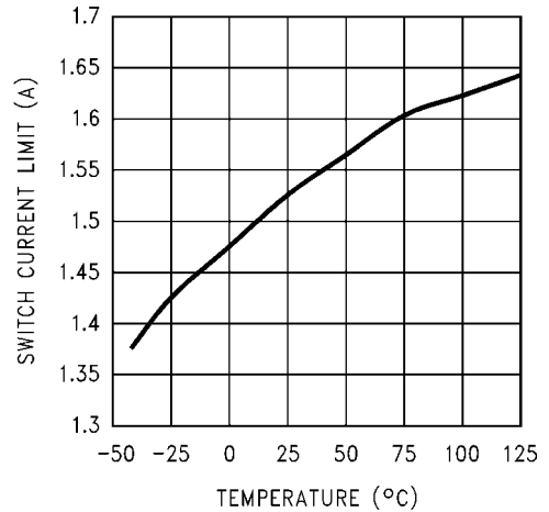
电流限值与温度的关系曲线
