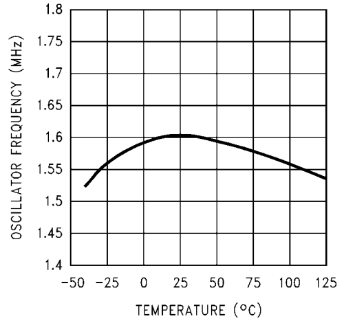
振荡器频率与温度的关系曲线
