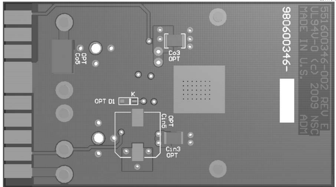
图1.评估印刷电路板顶部和底部视图
