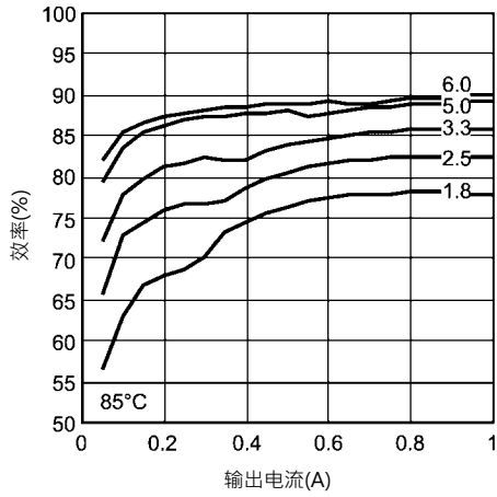
在85°C时20V输入效率
