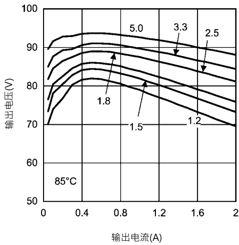
在85°C时8V输入效率
