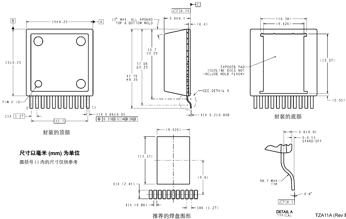
推荐的焊盘图形
