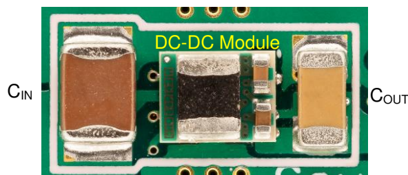
单面布局解决方案尺寸 24V 至 5V、0.5A 直流/直流转换器
