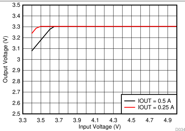
图 3. Dropout Voltage
