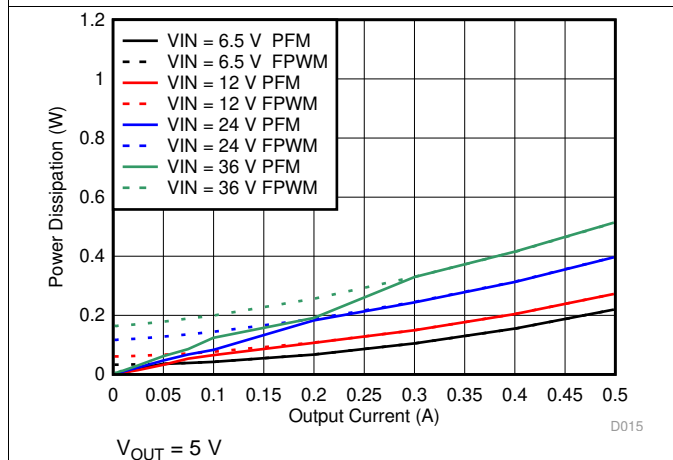
图 11. Power Dissipation
