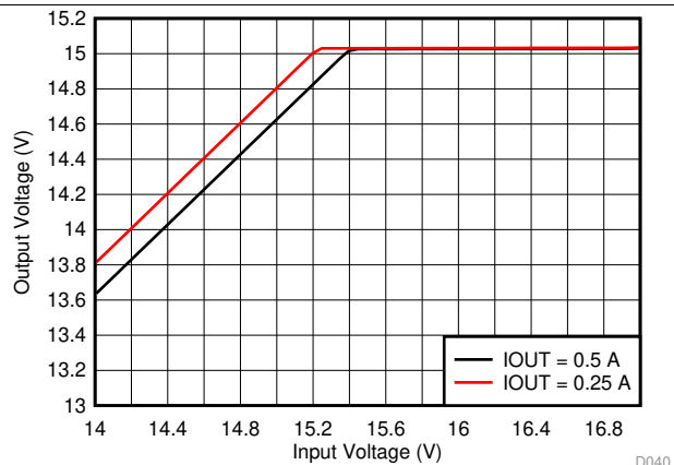
图 4. Dropout Voltage
