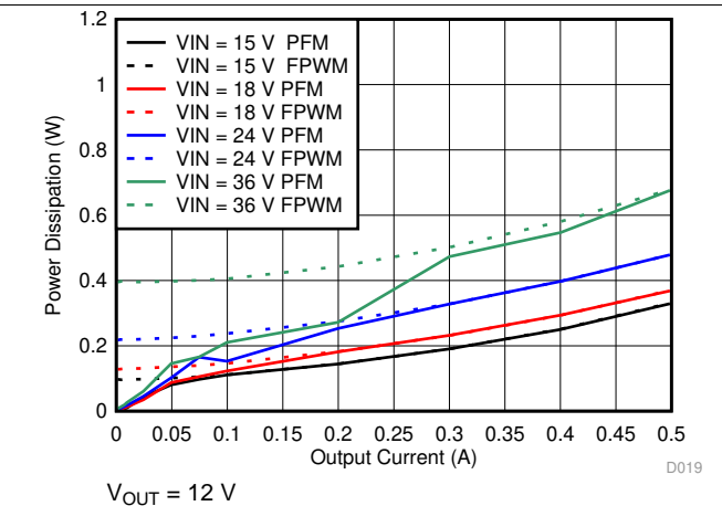
图 10. Power Dissipation
