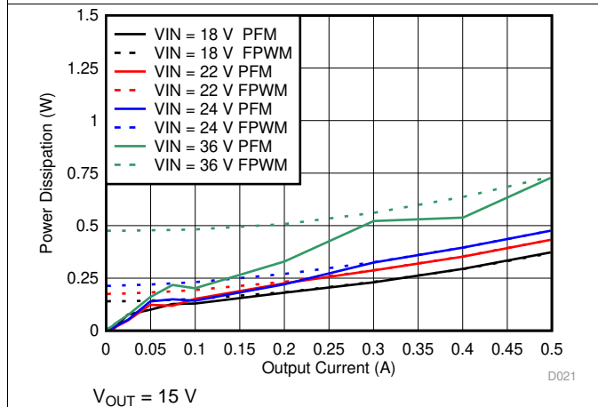
图 9. Power Dissipation
