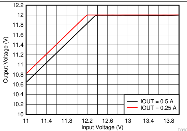
图 3. Dropout Voltage
