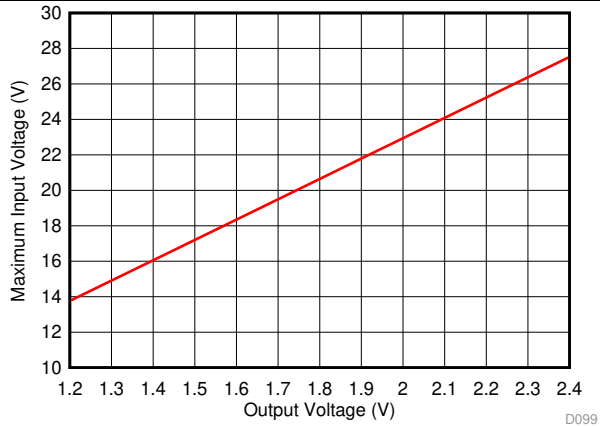
图 1. Maximum Input Voltage for V_{OUT} < 2.5\text{V}
