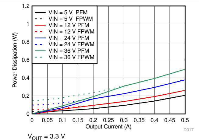
图 12. Power Dissipation
