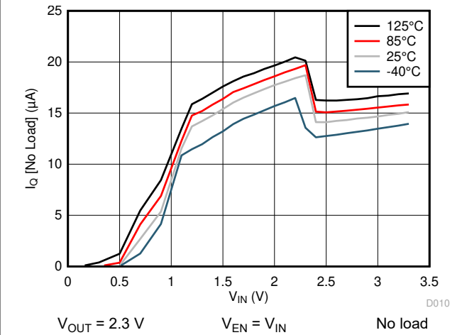
图 6-10. I_Q vs V_{IN}
