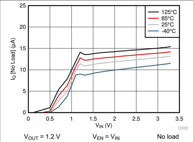
图 6-8. I_Q vs V_{IN}
