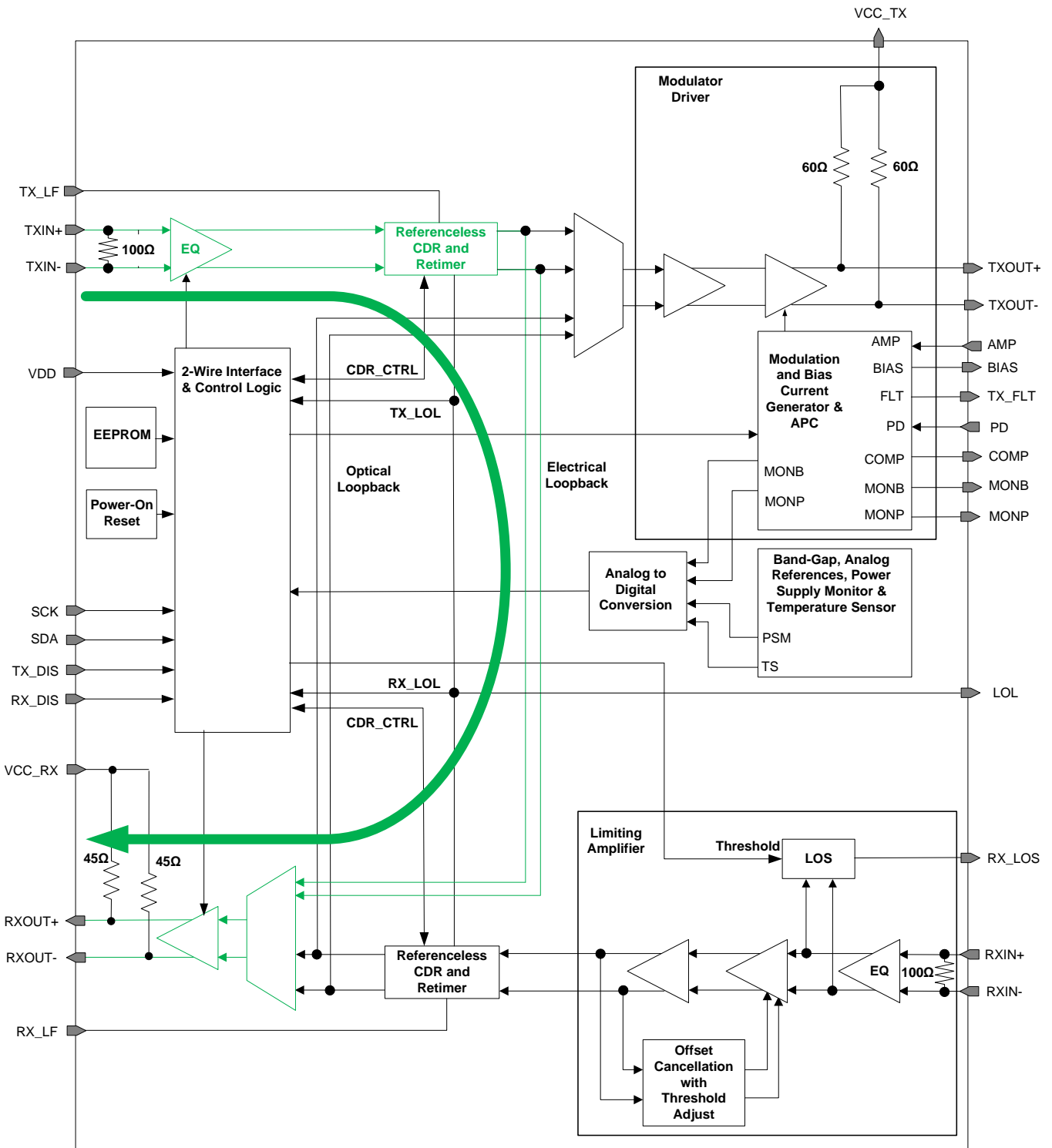
图 38. Electrical Loopback
