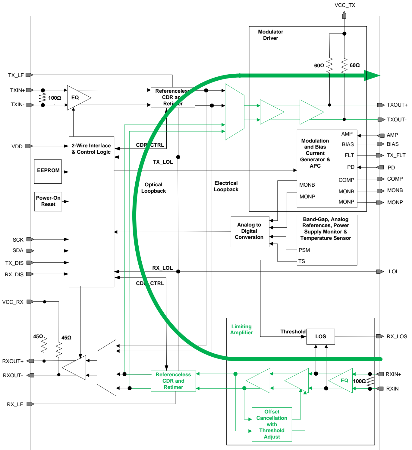
图 39. Optical Loopback
