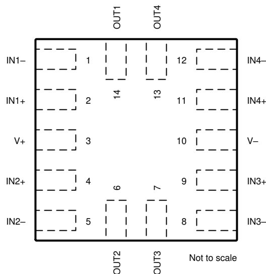
图 6-11. OPA4310 RUC 封装 14 引脚 X2QFN ( 顶视图 )
