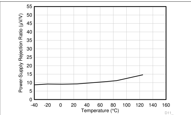
图 7-26. 直流 PSRR 与温度间的关系
