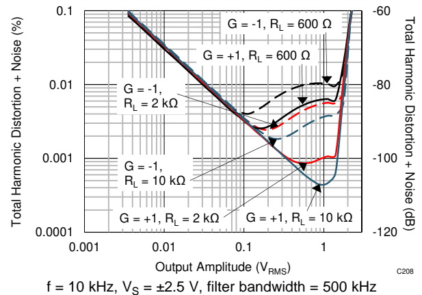
图 28. THD+N vs Amplitude
