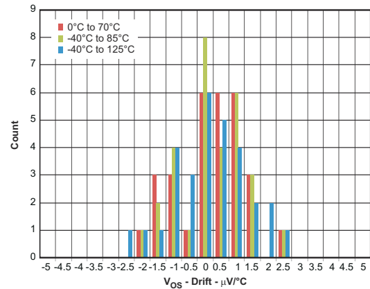
图 7-48. Input Offset Voltage Drift
