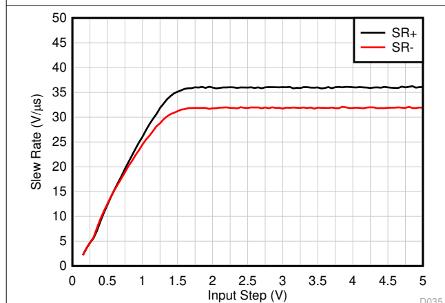
图 6-15. 压摆率与输入阶跃电压间的关系
