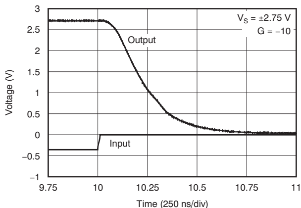
图 31. 正恢复时间
