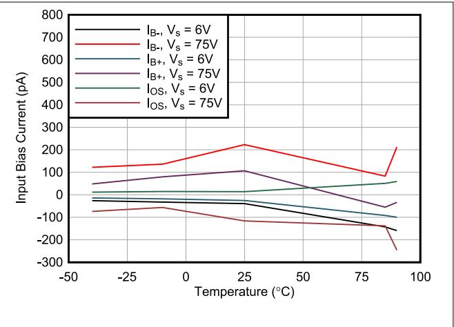
图 6-20. IB vs Temperature
