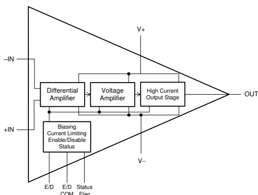
OPA455 方框图
