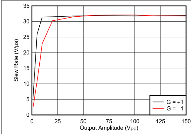
图 6-43. Slew Rate vs Output Step Size
