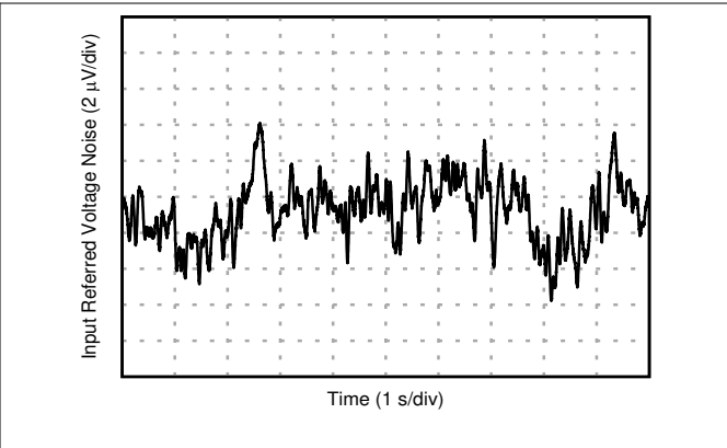
图 6-50. 0.1-Hz to 10-Hz Noise
