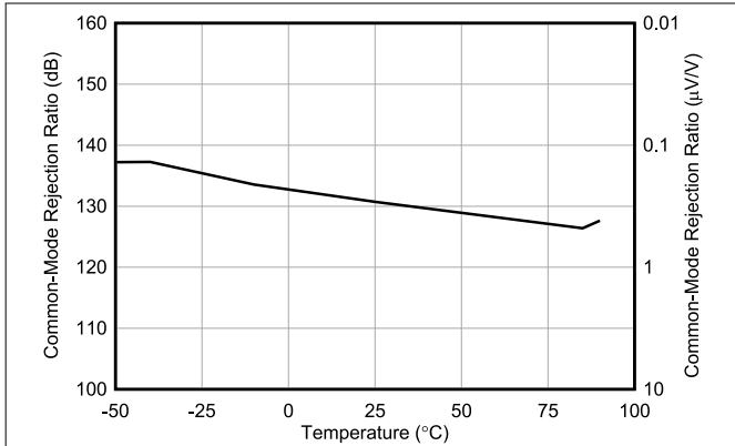
图 6-13. CMRR vs Temperature
