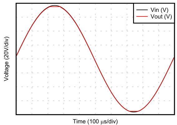
图 6-18. No Phase Reversal
