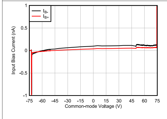
图 6-21. IB vs Common-Mode Voltage
