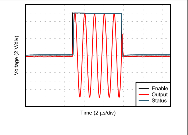
图 6-22. Enable Response
