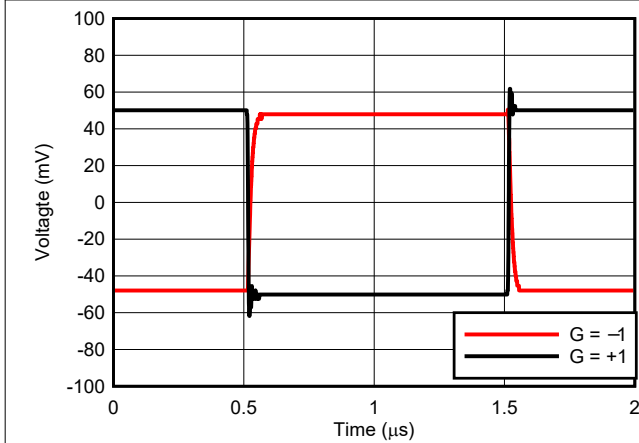
图 6-31. 正过载恢复
