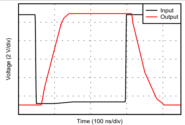
图 6-32. 负过载恢复
