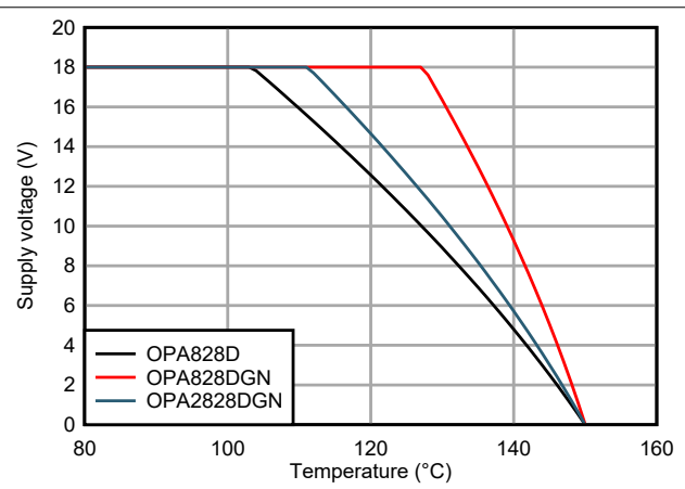
图 8-8. OPAx828 600Ω 负载热安全工作区
