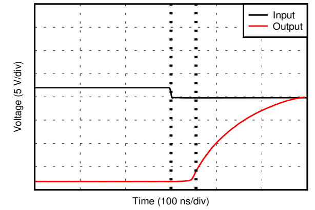
图 6-30. 无相位反转
