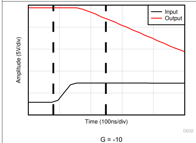
图 6-35. 正过载恢复
