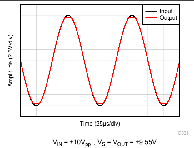
图 6-34. 无相位反转
