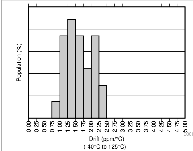
图 7-1. Temperature Drift
