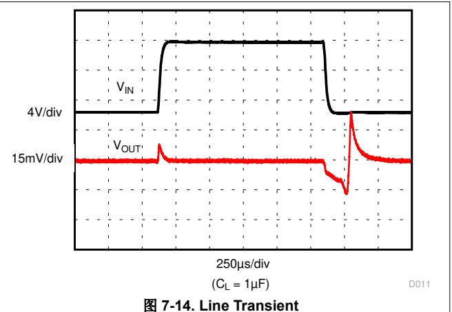
图 7-14. Line Transient
