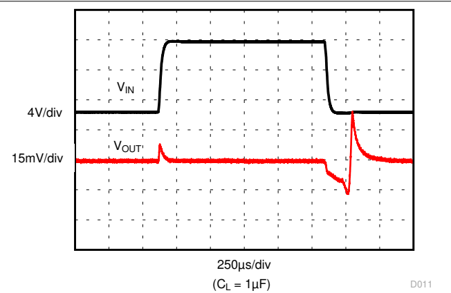
图 7-14. Line Transient
