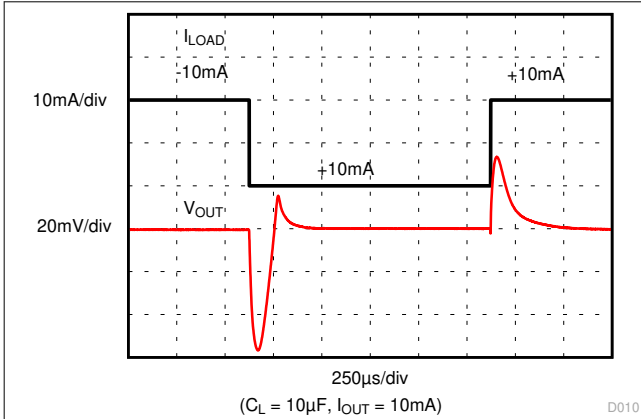
图 7-13. Load Transient
