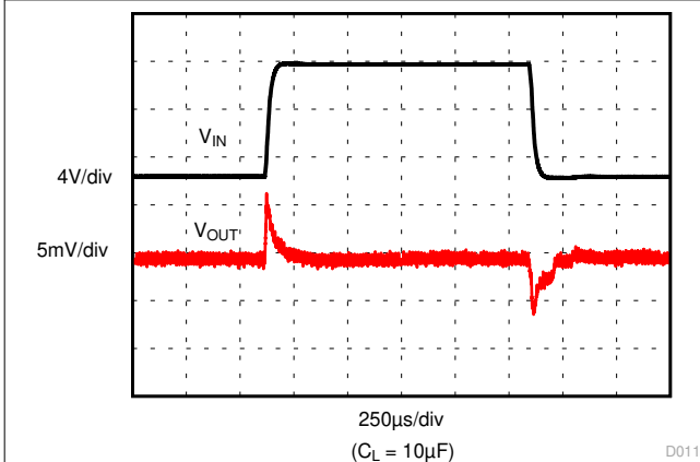
图 7-15. Line Transient
