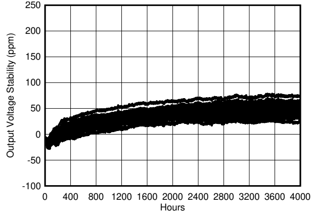
图 7-26. REF50xx 长期稳定性 (4000 小时)
