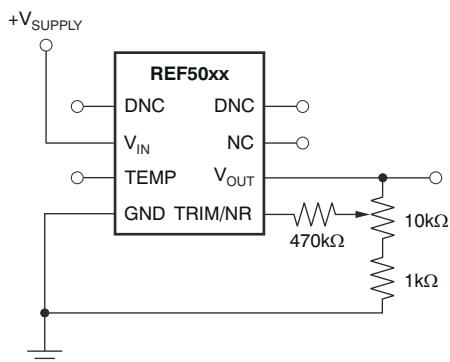
图 9-3. 使用 TRIM/NR 引脚进行 V_{\text{OUT}} 调节
