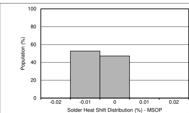
图 8-3. 焊接热移位分配 (%), VSSOP 封装
