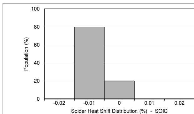
图 8-2. 焊接热移位分配 (%), SOIC 封装
