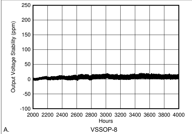
图 7-25. REF50xx 长期稳定性 (后 2000 小时)
