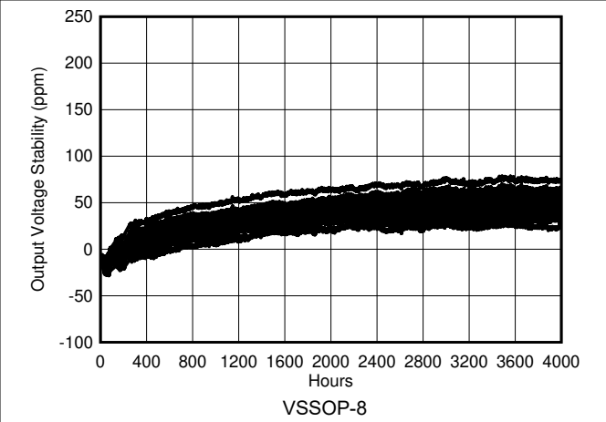
图 7-26. REF50xx 长期稳定性 (4000 小时)
