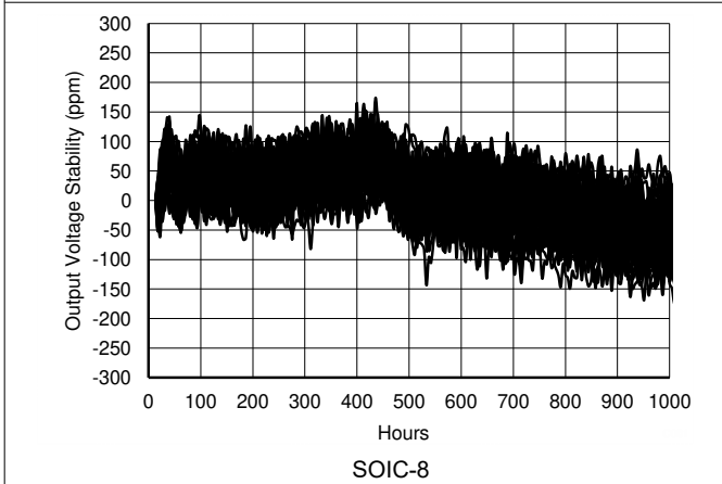
图 7-27. REF50xx 长期稳定性 (前 1000 小时)
