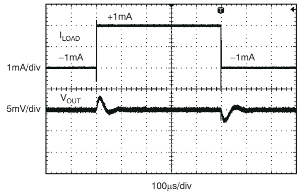
图 7-16. 负载瞬态
