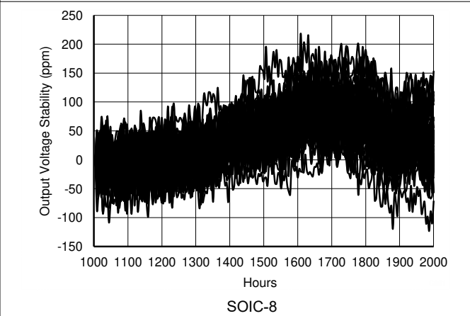
图 7-28. REF50xx 长期稳定性 (后 1000 小时)
