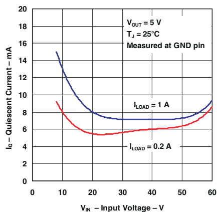
图 6-5. Quiescent Current
