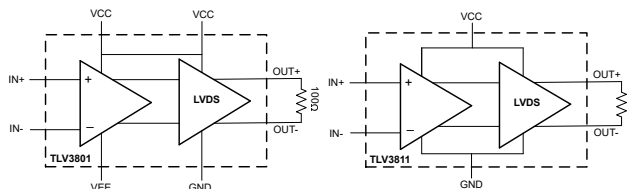
功能方框图
