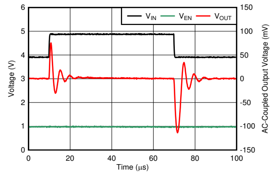
图 6-18. Line Transient
