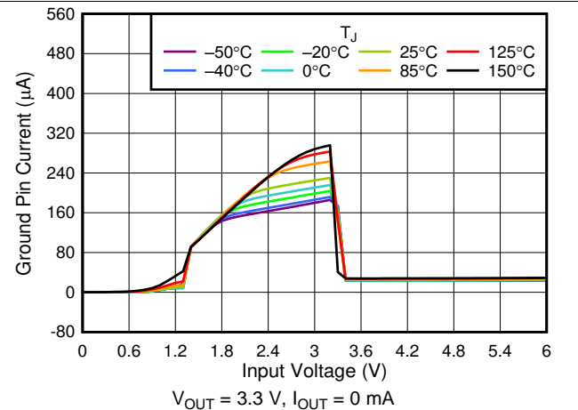
图 10. I_{GND} vs V_{IN}
