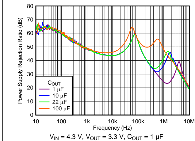
图 3. PSRR vs C_{OUT}
