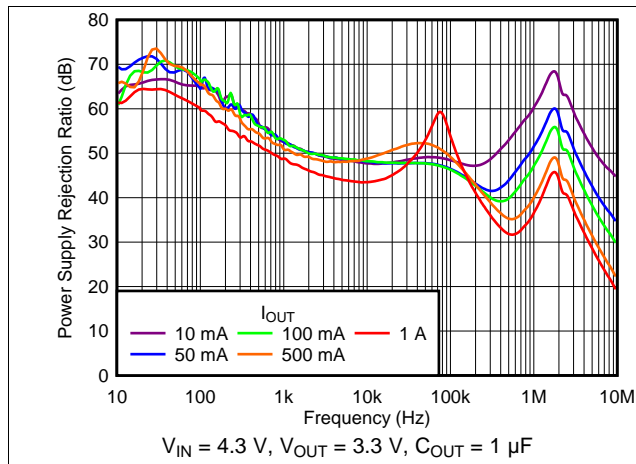
图 1. PSRR vs I_{OUT}
