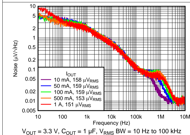
图 5. Output Spectral Noise Density
