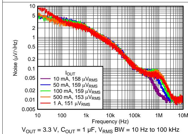
图 5. Output Spectral Noise Density
