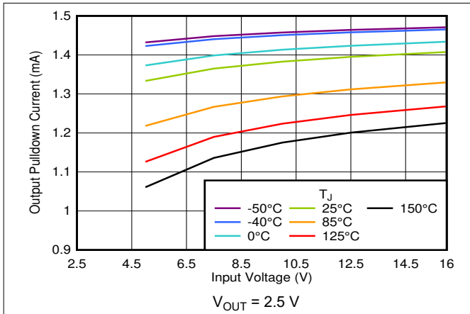
图 7-31. I_{PULLDOWN} vs V_{IN}
