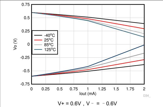
图 7-16. 输出电压与输出电流间的关系 (爪形)
