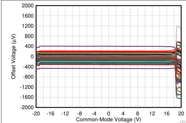
T_A = 125^\circ\text{C} 来自 74 个放大器的数据
