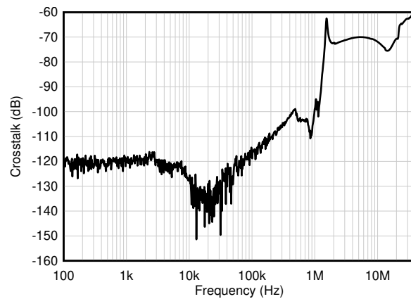
图 6-36. 通道隔离与频率间的关系
