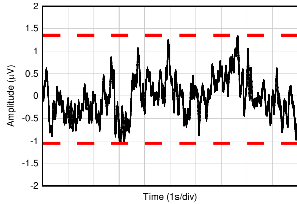
图 6-20. 0.1Hz 至 10Hz 噪声
