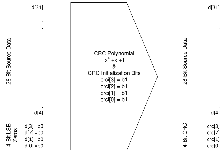
图 7-13. 4 位 CRC 计算
