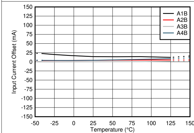
图 7-3. TMCS1101AxB-Q1 输入失调电流与温度间的关系
