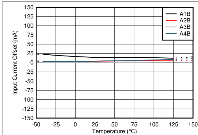
图 9-2. 整个温度范围内的失调误差漂移 (B 型号)
