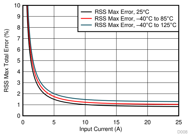
图 10-1. RSS 误差与输入电流间的关系
