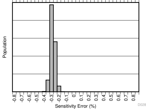
TMCS1101AxB-Q1
