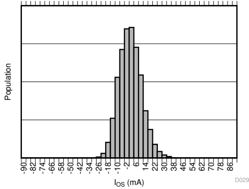
TMCS1101A1B-Q1
