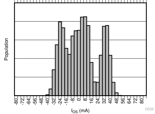
TMCS1101A2U-Q1
