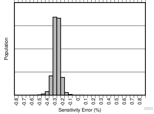
TMCS1101AxU-Q1
