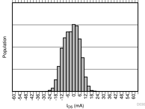
TMCS1101A2B-Q1
