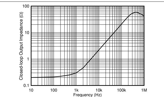
图 7-6. 输出阻抗与频率间的关系
