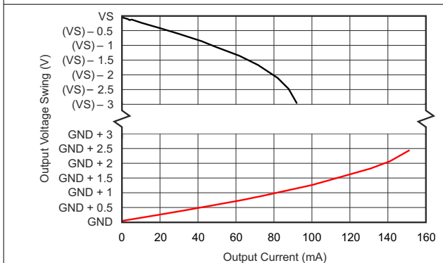
图 7-5. 输出摆幅与输出电流间的关系
