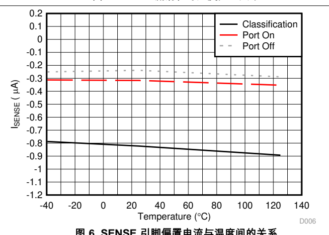
图 6. SENSE 引脚偏置电流与温度间的关系
