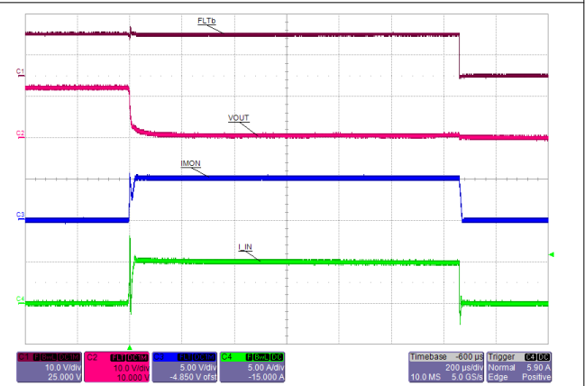
图 10-18. Hot Short: Latched - TPS25940L-Q1
