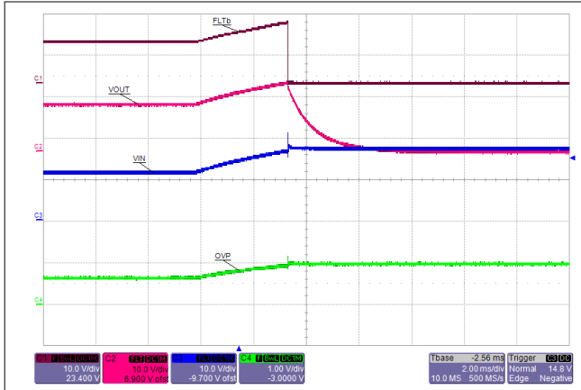
图 10-9. Overvoltage Shutdown
