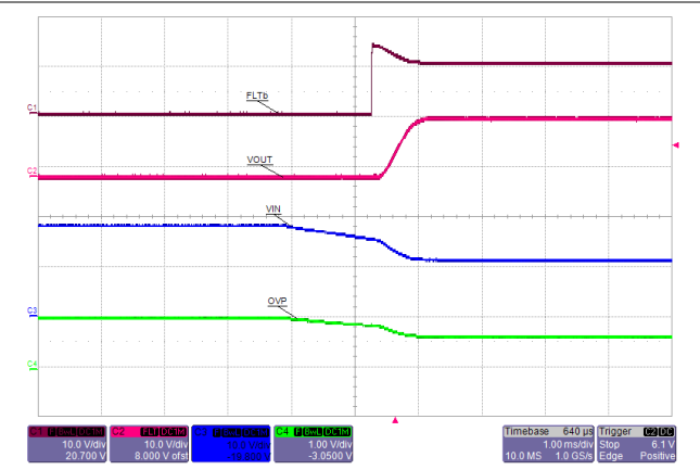
图 10-10. Overvoltage Recovery
