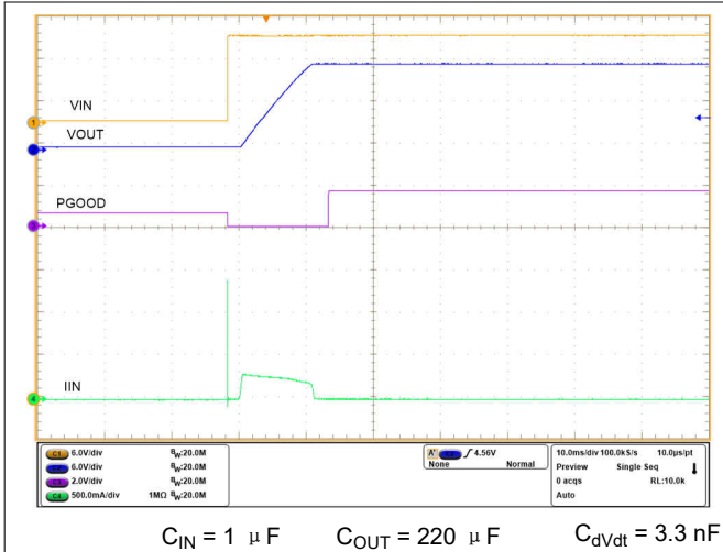
图 7-24. Hotplug
