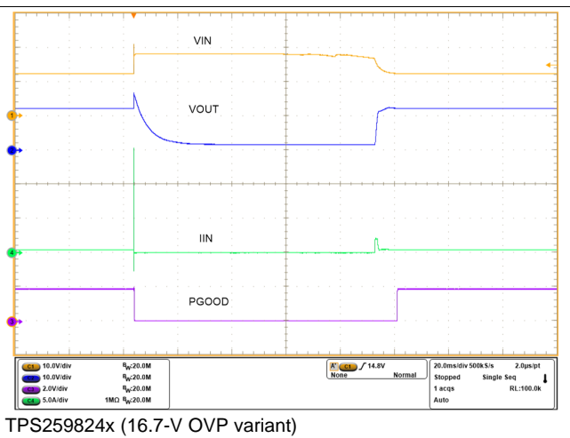
图 30. Overvoltage Protection
