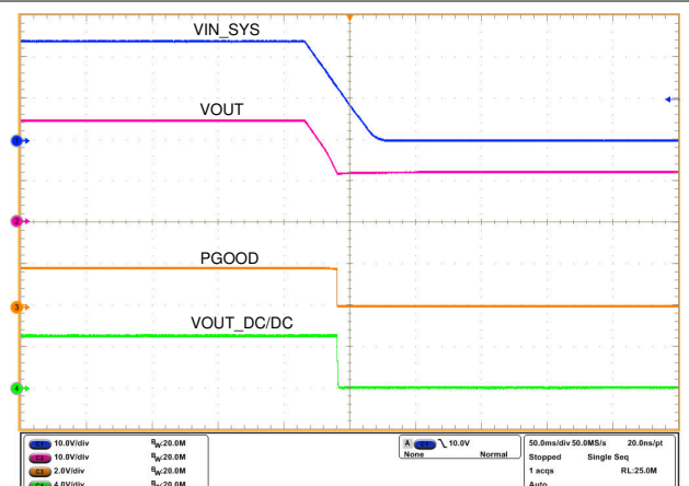
图 10-8. Power Down Response
