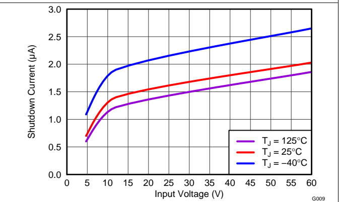
Figure 12. 关断电源电流 (I_IN) 与输入电压间的关系
