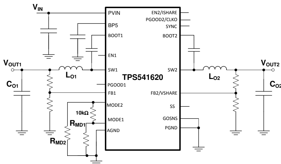
简化原理图 (双路输出)
