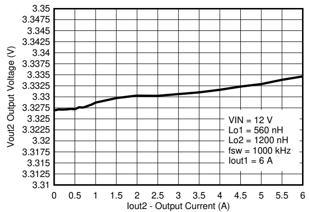
图 8-6. V_{OUT2} Load Regulation
