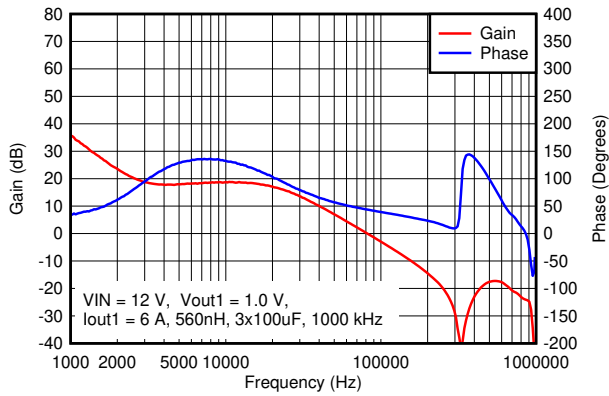
图 8-11. V_{OUT1} Bode Plot
