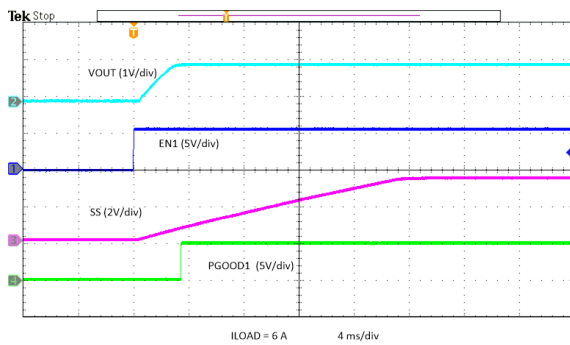
图 8-39. Power Up with EN
