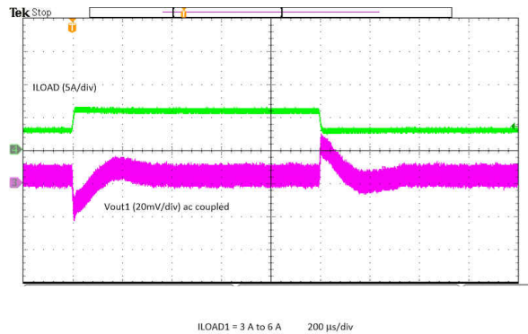
图 8-13. V_{OUT1} Load Transient
