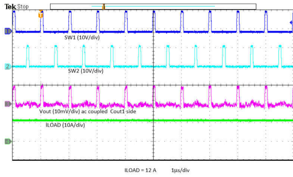
图 8-46. Output Ripple - 12-A Load
