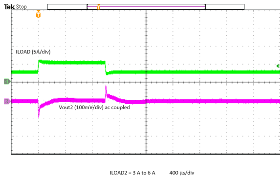
图 8-14. V_{OUT2} Load Transient
