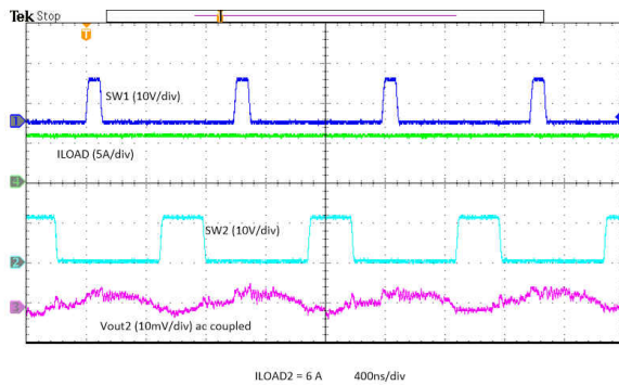
图 8-29. V_{OUT2} Output Ripple - 6-A Load
