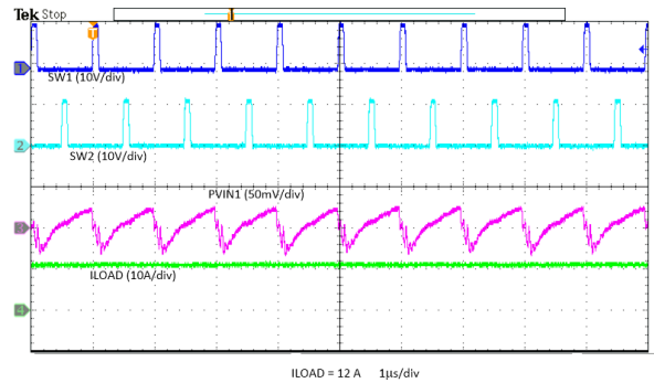
图 8-47. Input Ripple PVIN1 - 12-A Load
