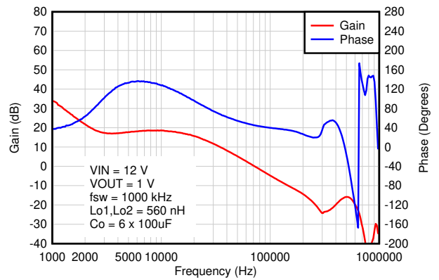
图 8-37. Bode Plot
