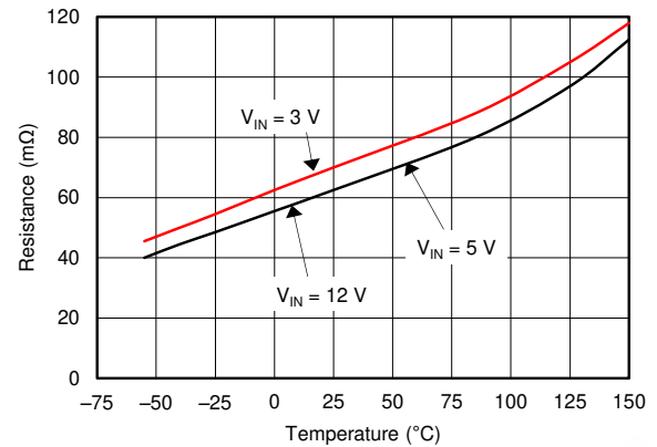
图 7-4. R_{DS(ON)} vs Temperature
